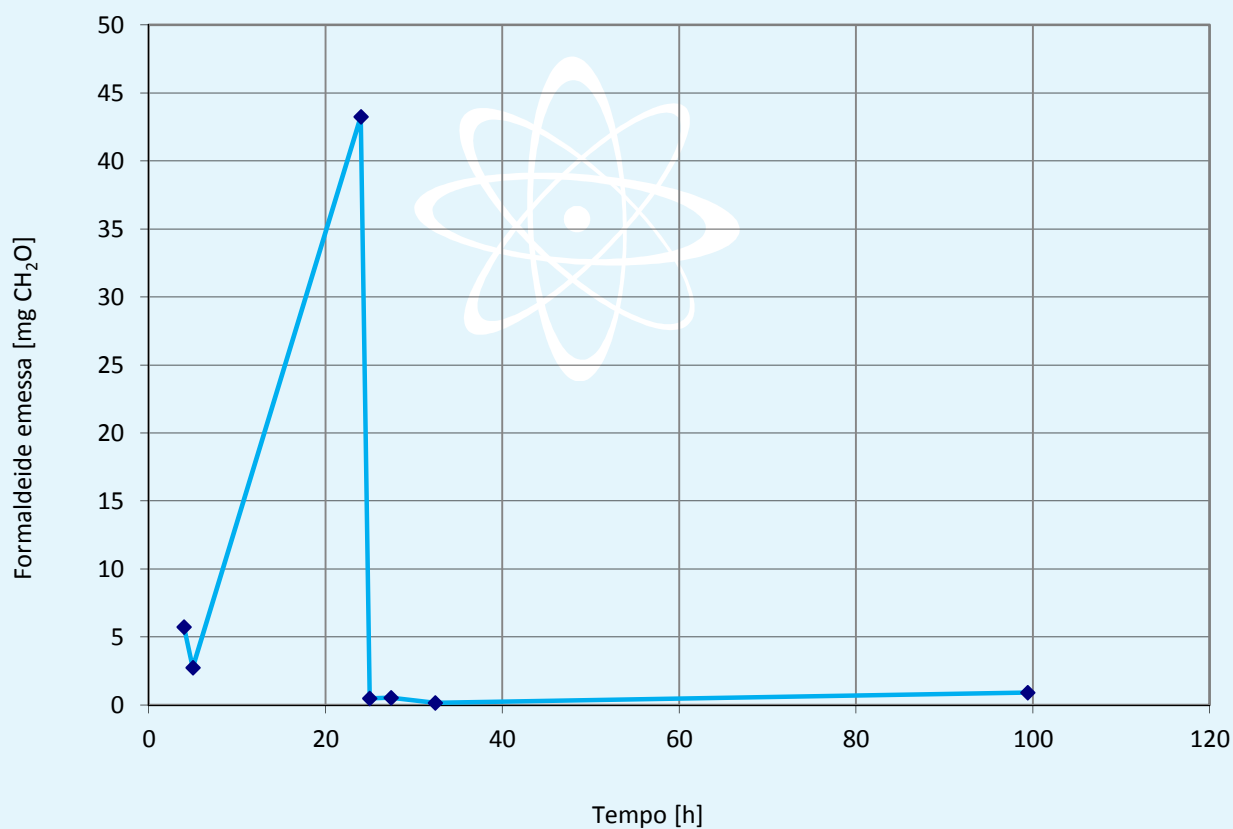
Grafico "1": espressione delle emissioni di formaldeide in funzione del tempo di campionamento.
