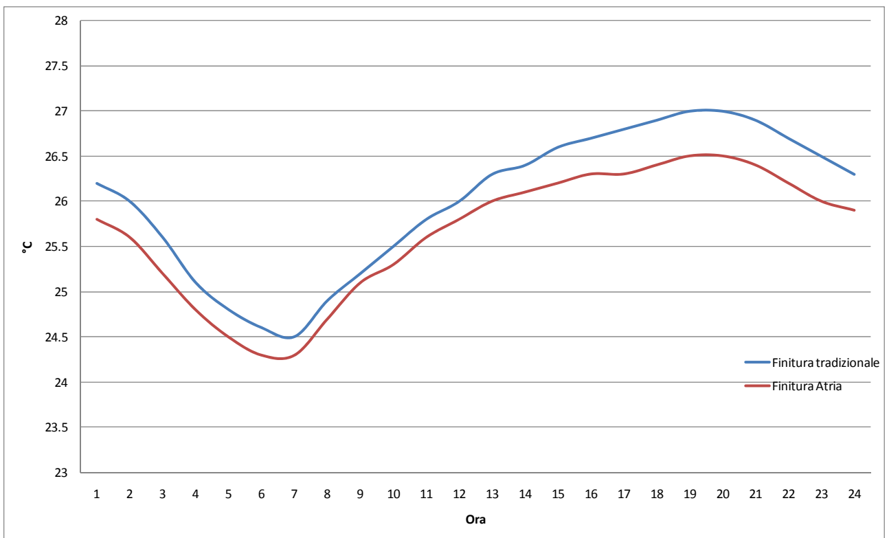
Figura 22 – Temperature interne superficiali nella parete EST nel caso di applicazione della finitura Atria Termica e della finitura tradizionale (giornata estiva)
