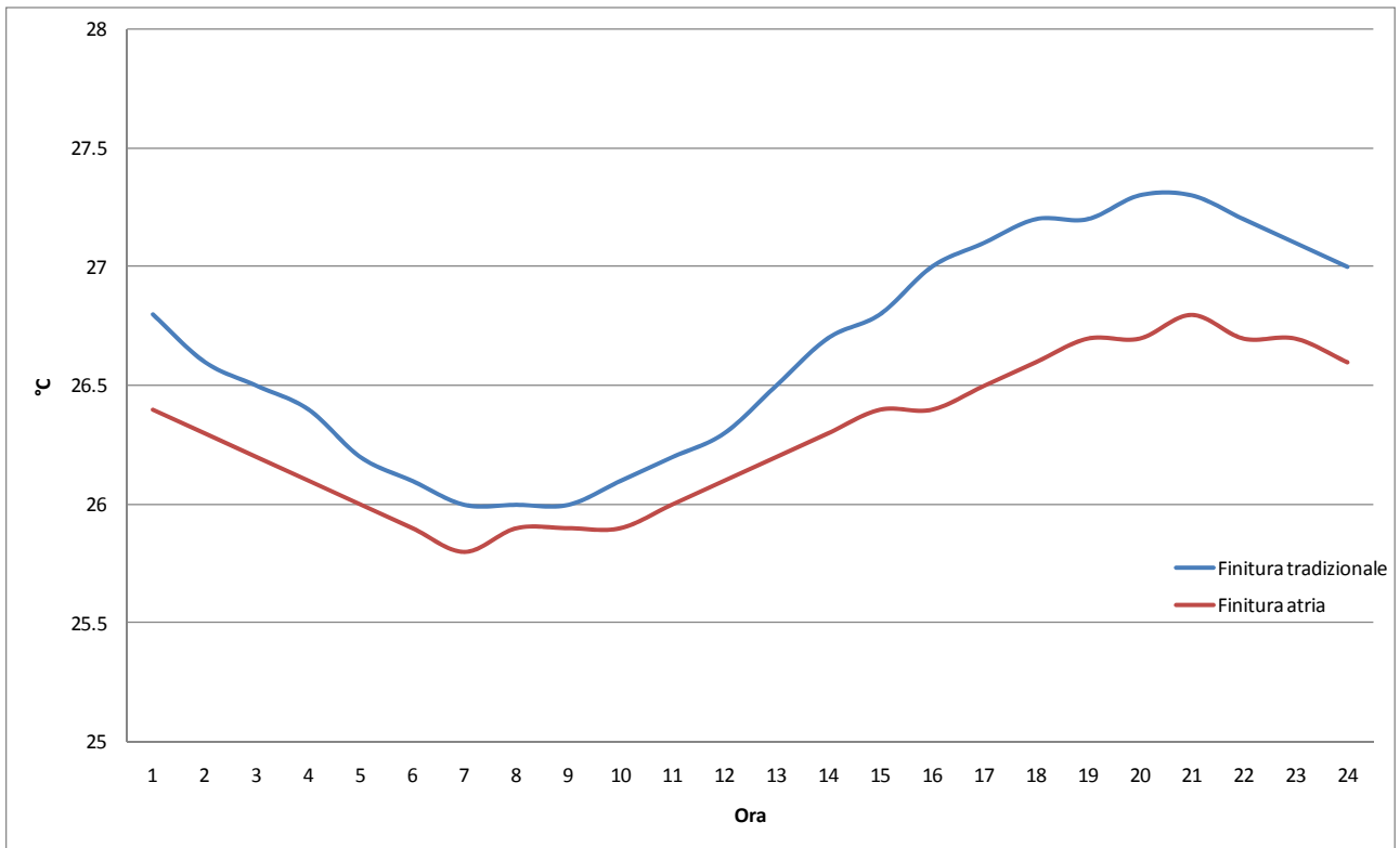
Figura 11 – Temperature interne superficiali nella parete SUD nel caso di applicazione della finitura Atria Thermica e della finitura tradizionale (giornata estiva)
