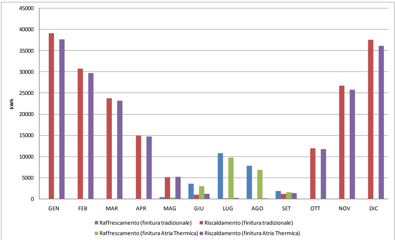
Figura 20 – Domanda di energia nel caso di “palazzina”: finitura Atria Thermica e finitura tradizionale
