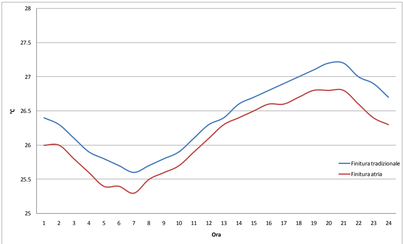
Figura 4 – Temperature interne superficiali nella parete SUD nel caso di applicazione della finitura Atria Thermica e della finitura tradizionale (giornata estiva)
