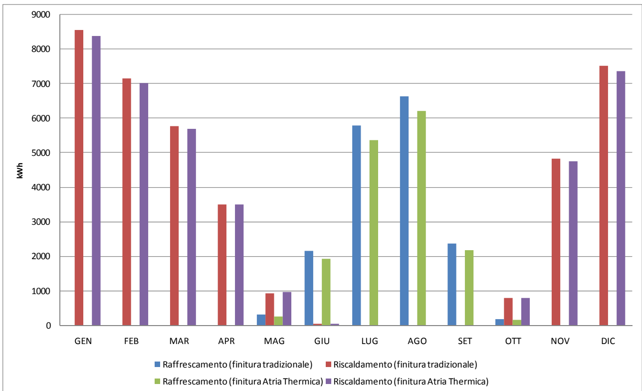
Figura 8 – Domanda di energia nel caso di “edificio a schiera”: finitura Atria Thermica e finitura tradizionale
