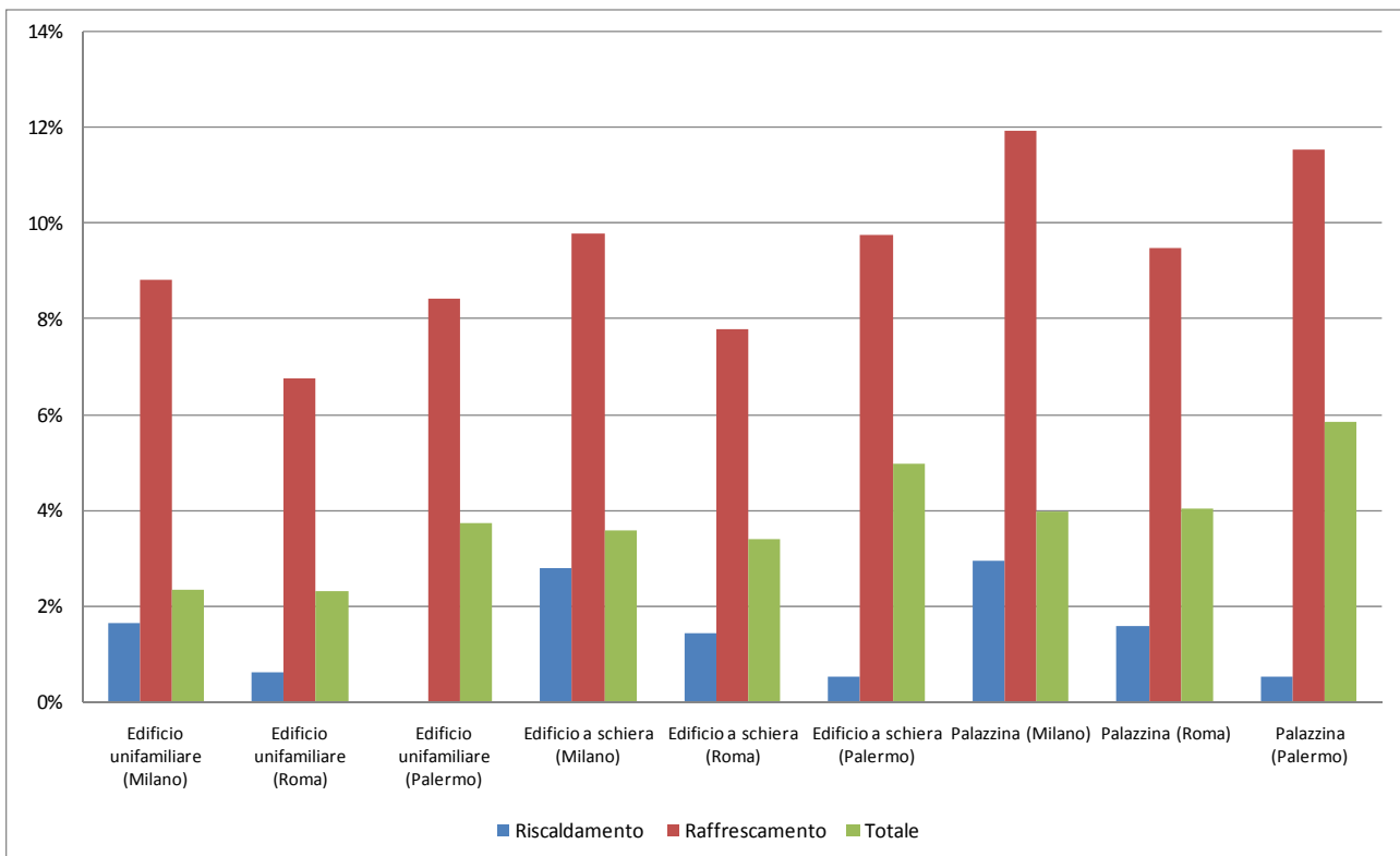
Figura 30 – Differenza tra domanda di energia per riscaldamento, raffrescamento e totale nel caso di applicazione di finitura Atria Thermica e di finitura tradizionale
