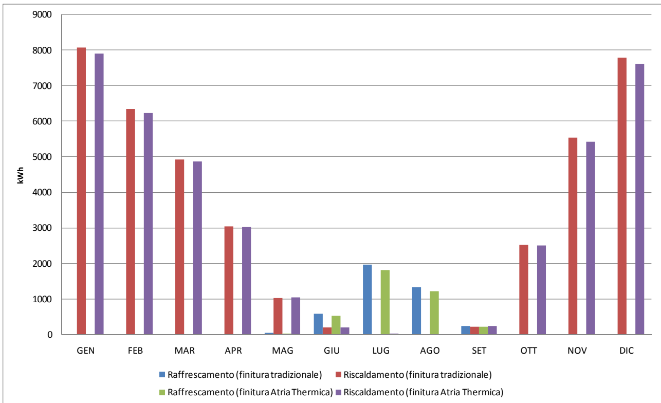
Figura 6 – Domanda di energia nel caso di “villetta unifamiliare”: finitura Atria Thermica e finitura tradizionale
