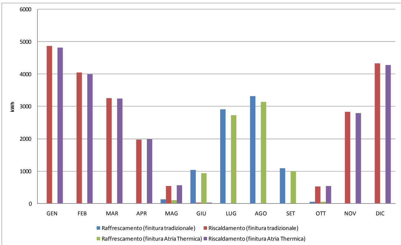
Figura 1 – Domanda di energia nel caso di “villetta unifamiliare”: finitura Atria Thermica e finitura tradizionale
