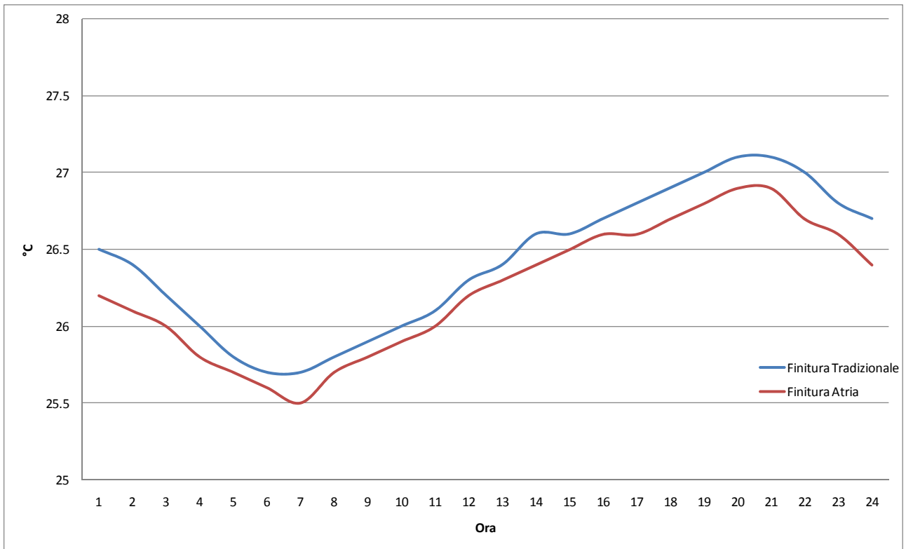
Figura 16 – Temperature interne superficiali nella parete NORD nel caso di applicazione della finitura Atria Termica e della finitura tradizionale (giornata estiva)
