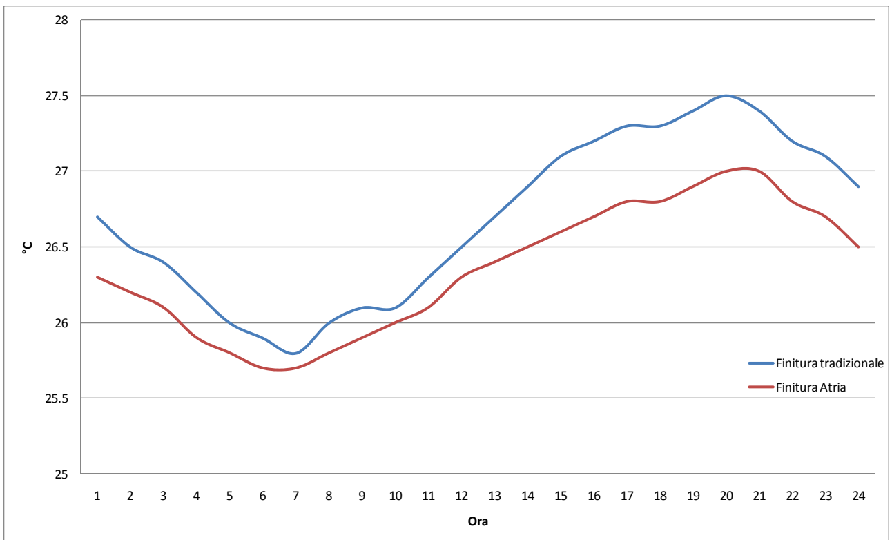
Figura 10 – Temperature interne superficiali nella parete EST nel caso di applicazione della finitura Atria Termica e della finitura tradizionale (giornata estiva)
