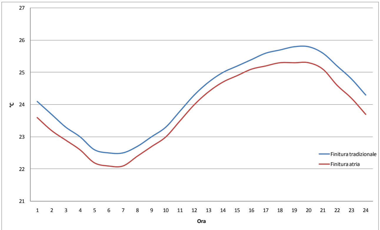
Figura 28 – Temperature interne superficiali nella parete SUD nel caso di applicazione della finitura Atria Termica e della finitura tradizionale (giornata estiva)
