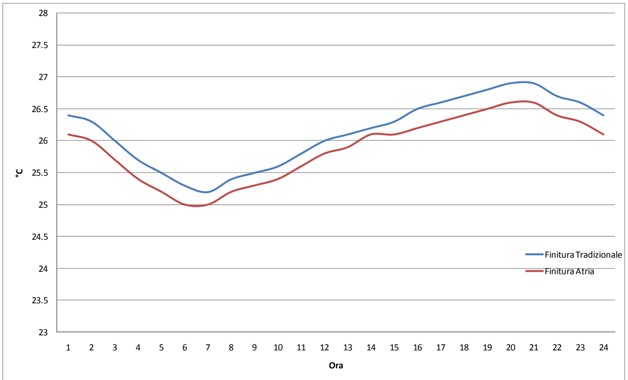
Figura 21 – Temperature interne superficiali nella parete NORD nel caso di applicazione della finitura Atria Termica e della finitura tradizionale (giornata estiva)
