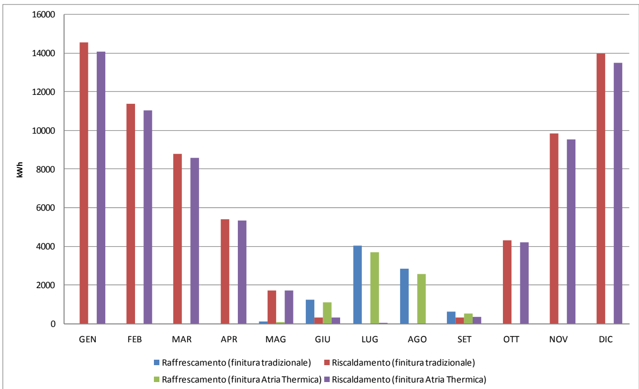
Figura 13 – Domanda di energia nel caso di “edificio a schiera”: finitura Atria Thermica e finitura tradizionale
