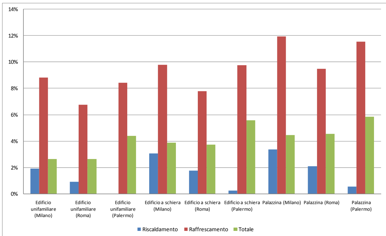
Figura 31 – Differenza tra domanda di energia per riscaldamento (periodi di riscaldamento fissati dal DPR 412/93), raffrescamento e totale nel caso di applicazione di finitura Atria Thermica e di finitura tradizionale
