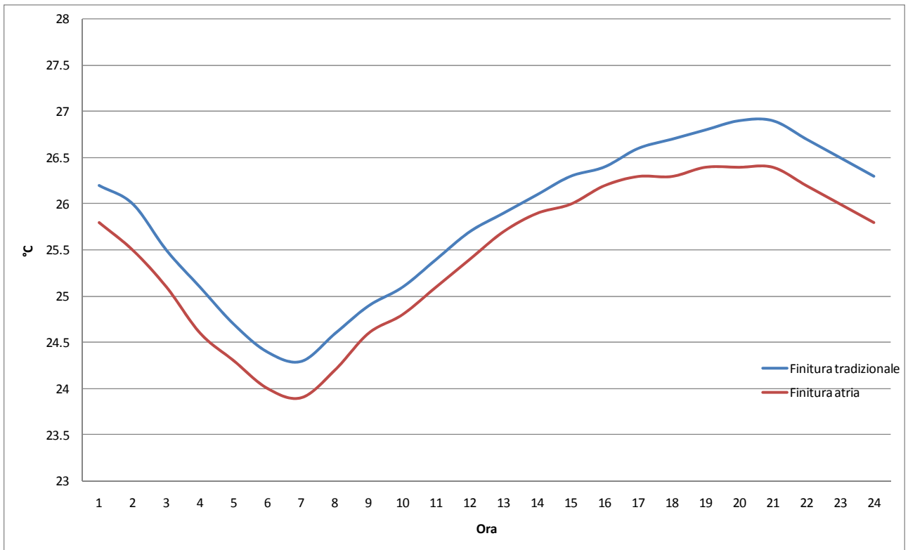
Figura 23 – Temperature interne superficiali nella parete SUD nel caso di applicazione della finitura Atria Termica e della finitura tradizionale (giornata estiva)
