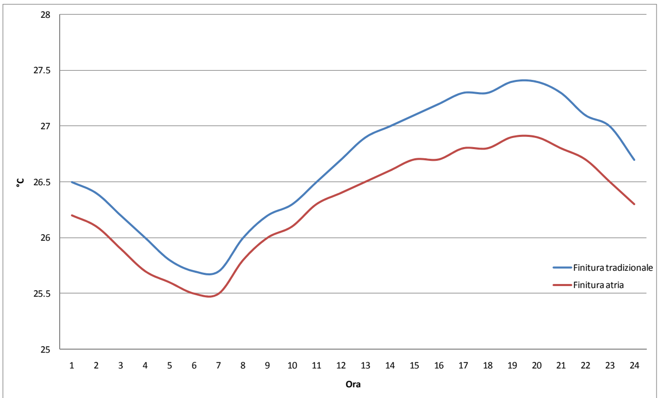
Figura 5 – Temperature interne superficiali nella parete OVEST nel caso di applicazione della finitura Atria Thermica e della finitura tradizionale (giornata estiva)
