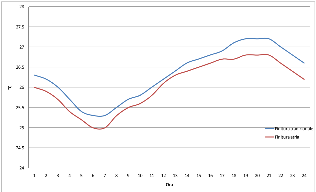
Figura 18 – Temperature interne superficiali nella parete SUD nel caso di applicazione della finitura Atria Termica e della finitura tradizionale (giornata estiva)
