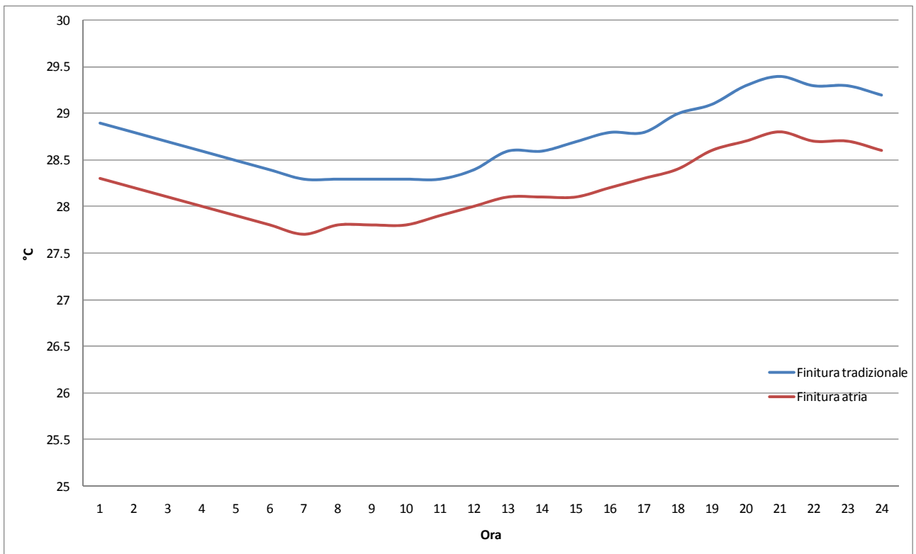
Figura 12 – Temperature interne superficiali nella parete OVEST nel caso di applicazione della finitura Atria Thermica e della finitura tradizionale (giornata estiva)
