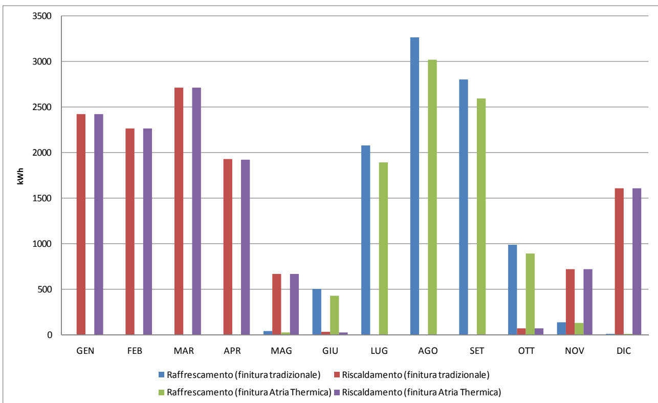
Figura 7 – Domanda di energia nel caso di “villetta unifamiliare”: finitura Atria Thermica e finitura tradizionale
