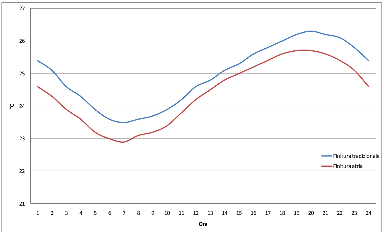
Figura 29 – Temperature interne superficiali nella parete OVEST nel caso di applicazione della finitura Atria Termica e della finitura tradizionale (giornata estiva)
