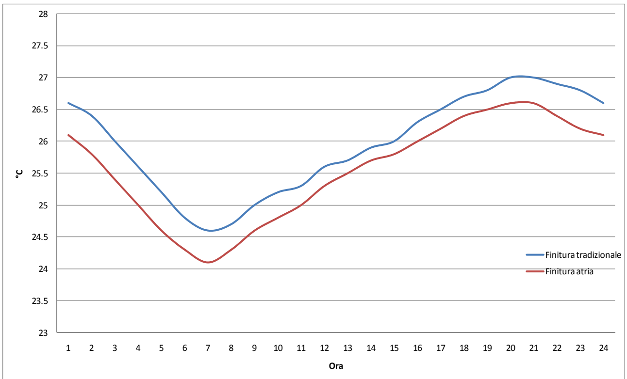
Figura 24 – Temperature interne superficiali nella parete OVEST nel caso di applicazione della finitura Atria Termica e della finitura tradizionale (giornata estiva)
