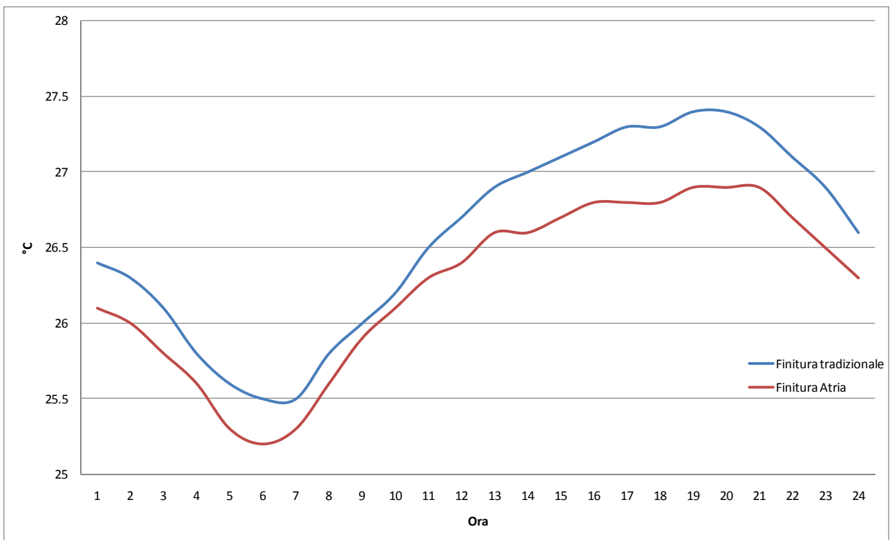
Figura 17 – Temperature interne superficiali nella parete EST nel caso di applicazione della finitura Atria Termica e della finitura tradizionale (giornata estiva)
