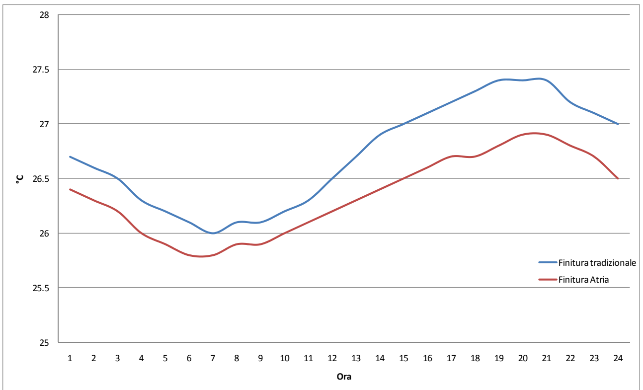
Figura 3 – Temperature interne superficiali nella parete EST nel caso di applicazione della finitura Atria Termica e della finitura tradizionale (giornata estiva)
