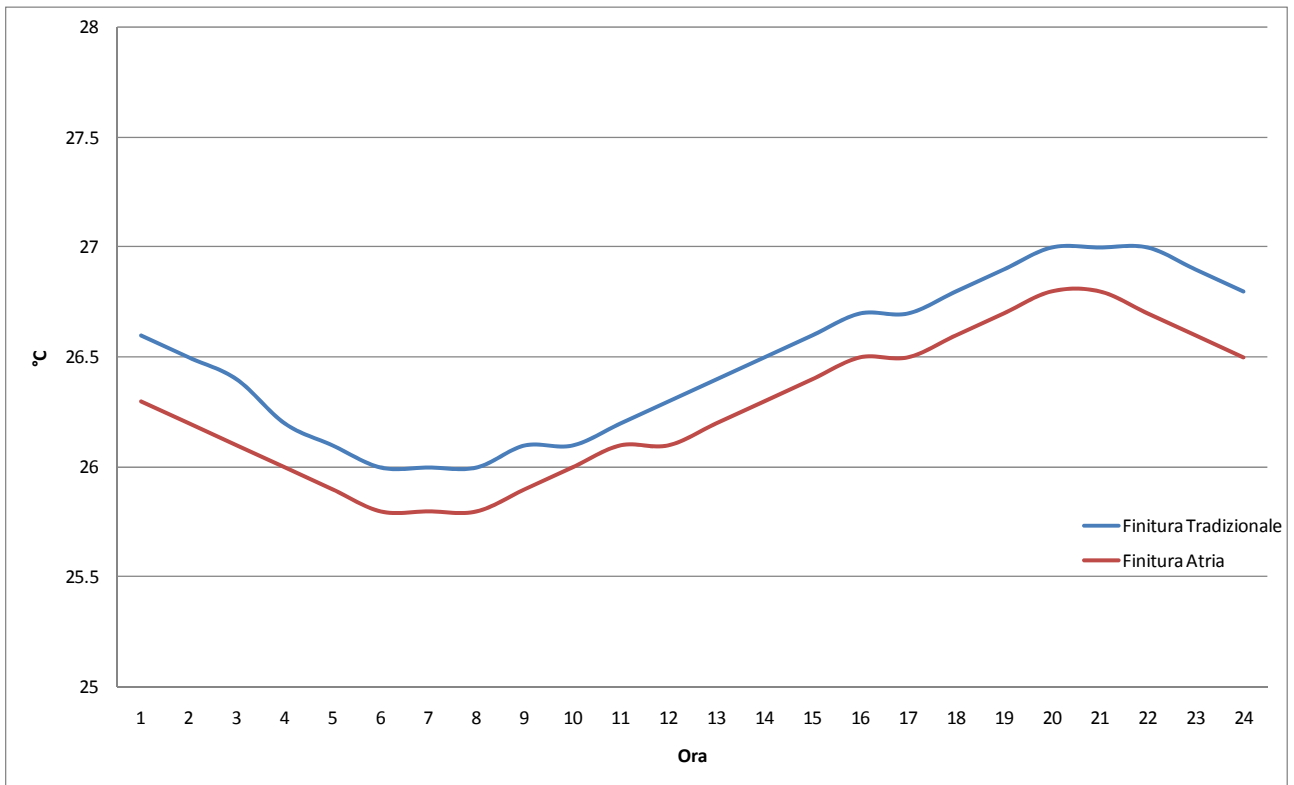
Figura 2 – Temperature interne superficiali nella parete NORD nel caso di applicazione della finitura Atria Termica e della finitura tradizionale (giornata estiva)
