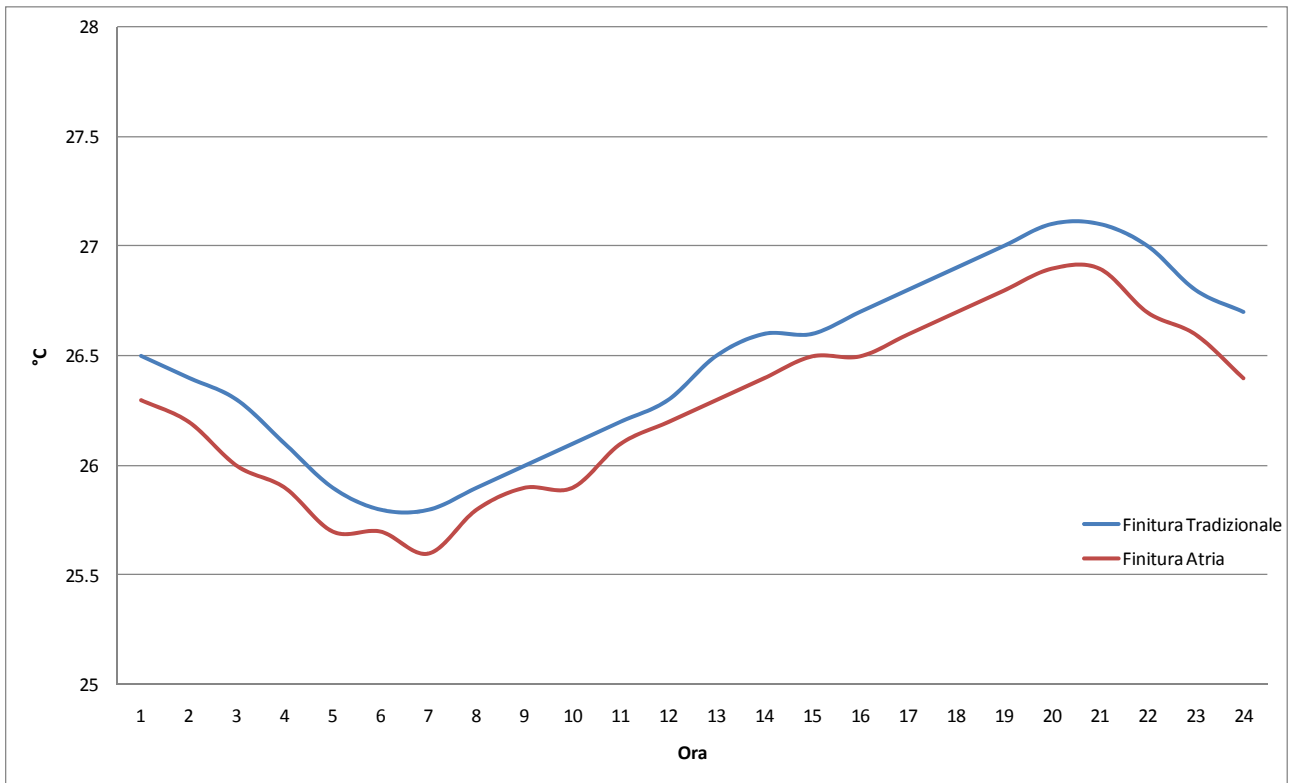
Figura 9 – Temperature interne superficiali nella parete NORD nel caso di applicazione della finitura Atria Termica e della finitura tradizionale (giornata estiva)
