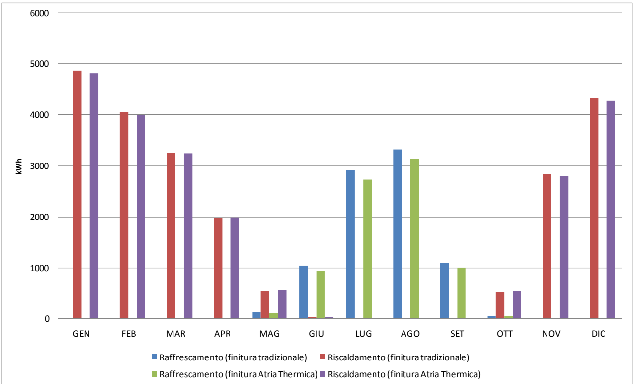
Figura 15 – Domanda di energia nel caso di “palazzina”: finitura Atria Thermica e finitura tradizionale
