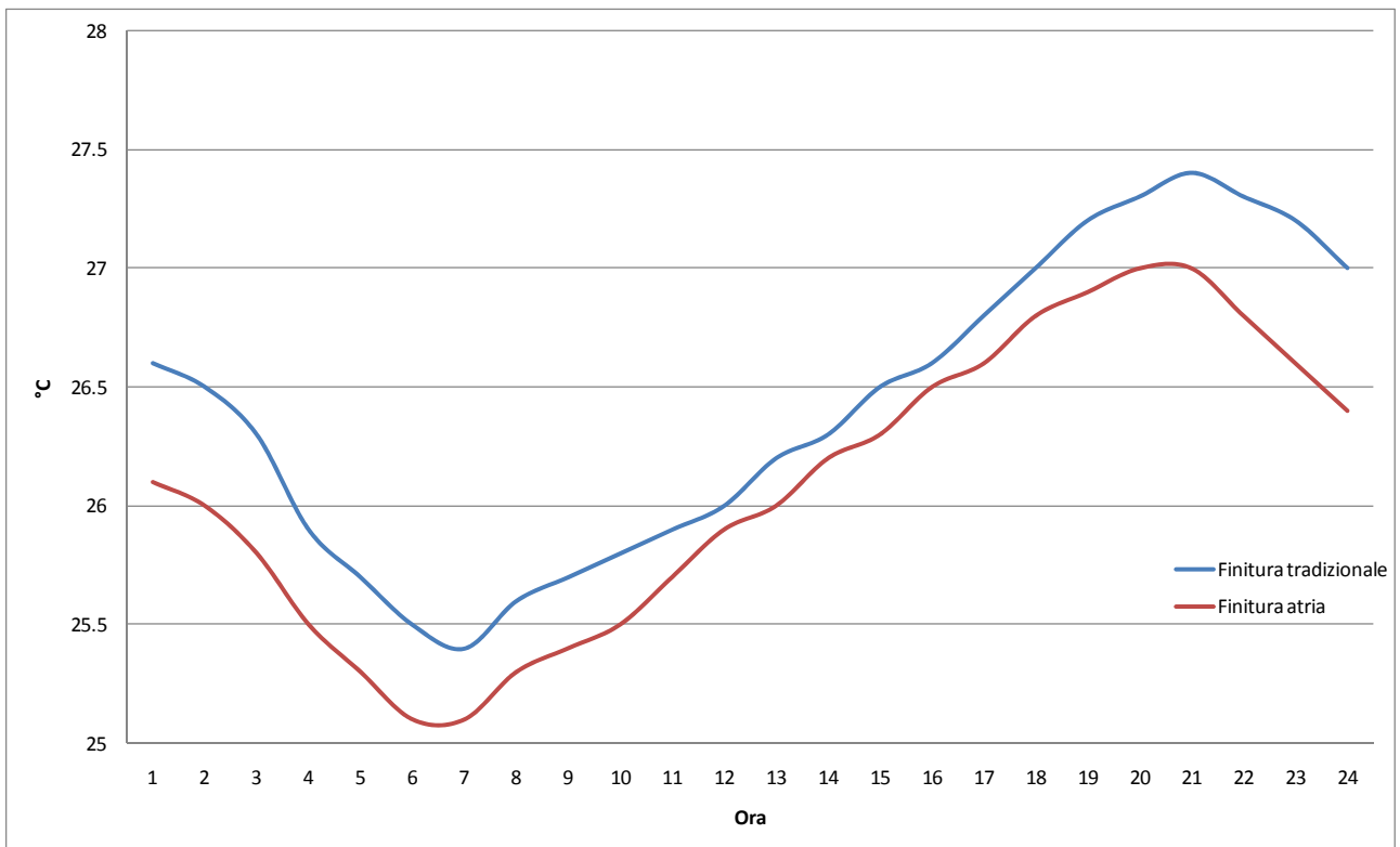
Figura 19 – Temperature interne superficiali nella parete OVEST nel caso di applicazione della finitura Atria Termica e della finitura tradizionale (giornata estiva)
