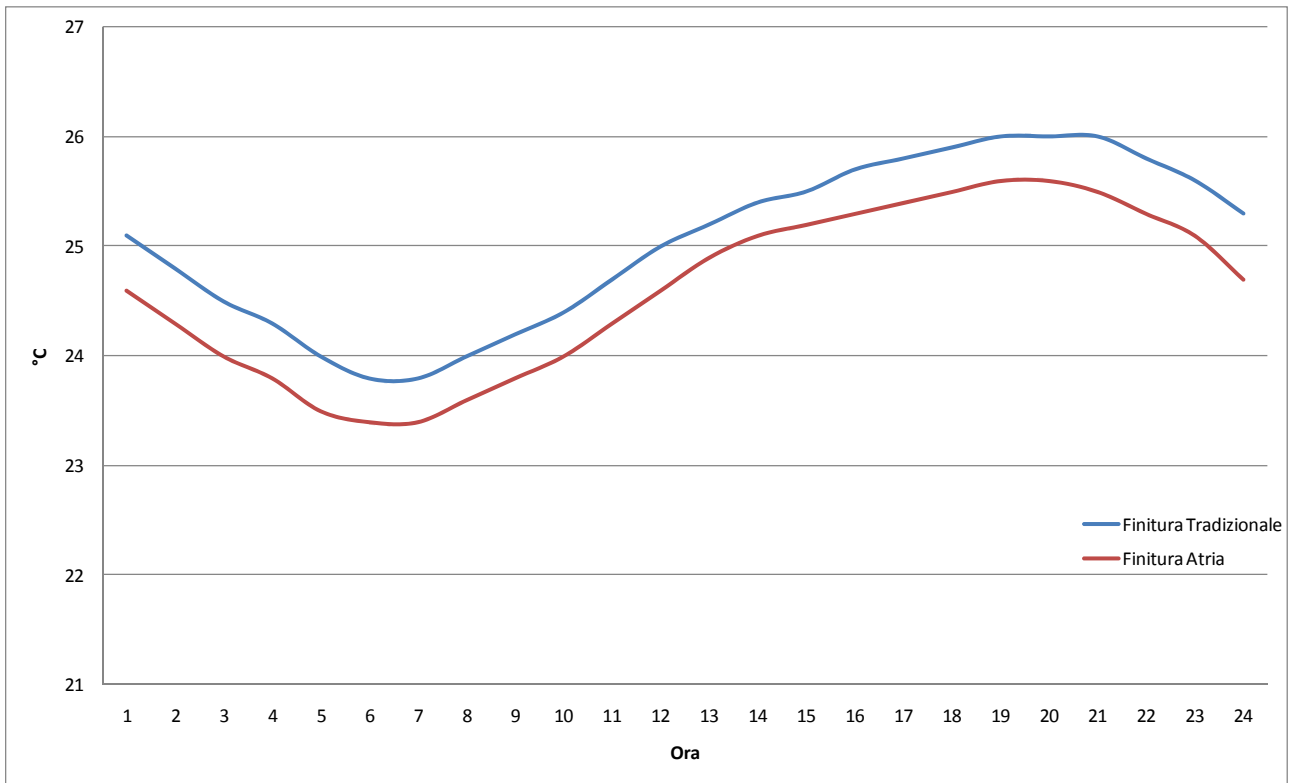
Figura 26 – Temperature interne superficiali nella parete NORD nel caso di applicazione della finitura Atria Termica e della finitura tradizionale (giornata estiva)
