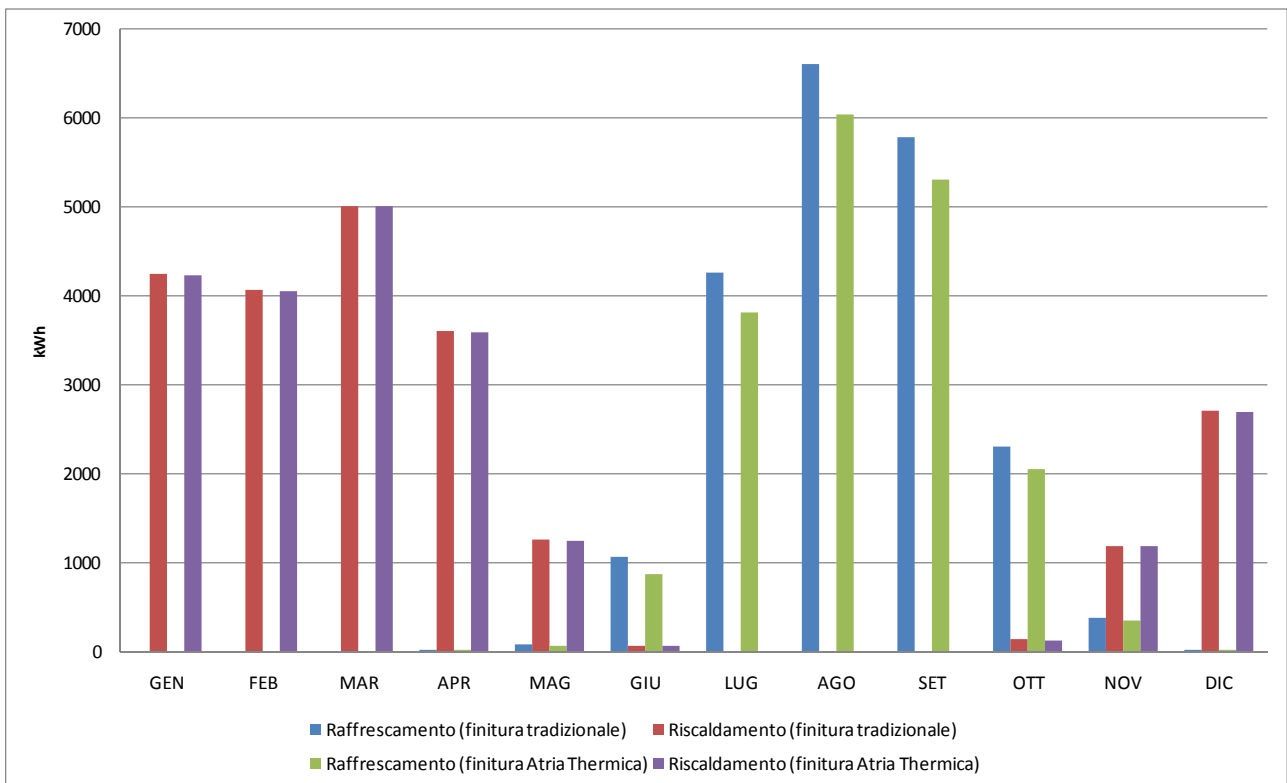
Figura 14 – Domanda di energia nel caso di “edificio a schiera”: finitura Atria Thermica e finitura tradizionale
