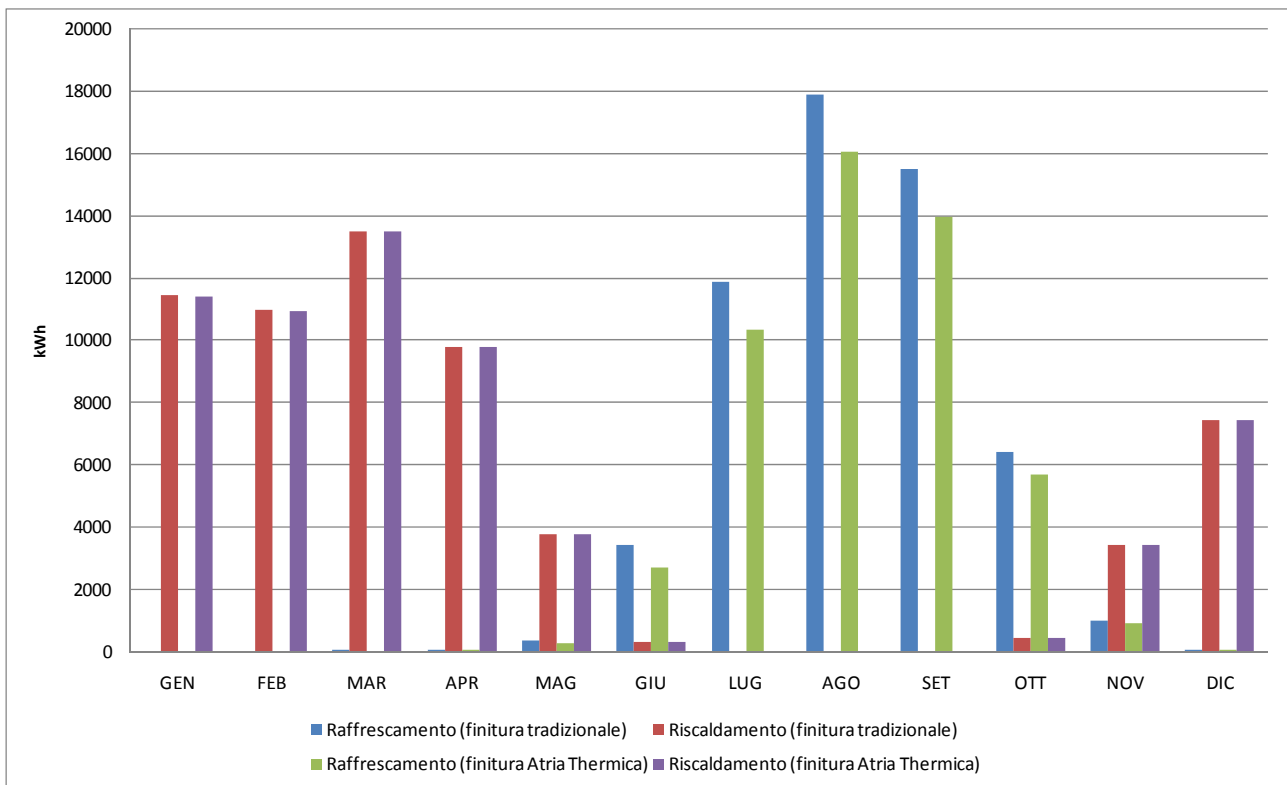
Figura 25 – Domanda di energia nel caso di “palazzina”: finitura Atria Thermica e finitura tradizionale
