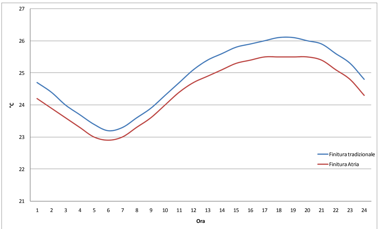
Figura 27 – Temperature interne superficiali nella parete EST nel caso di applicazione della finitura Atria Termica e della finitura tradizionale (giornata estiva)
